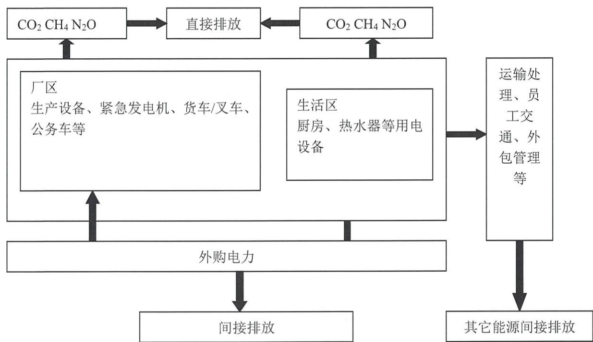
图-1 运行边界示意图
